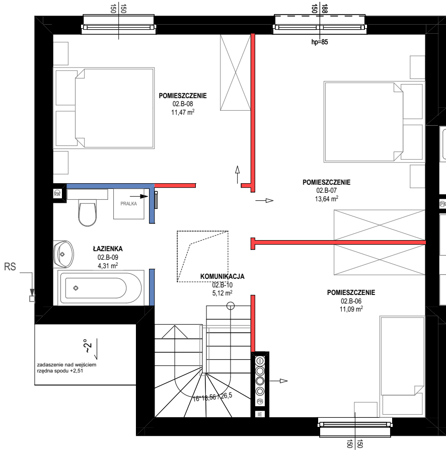
RZUT 1 PIĘTRA
