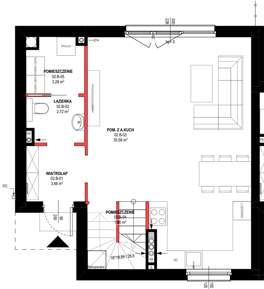
RZUT PARTERU
